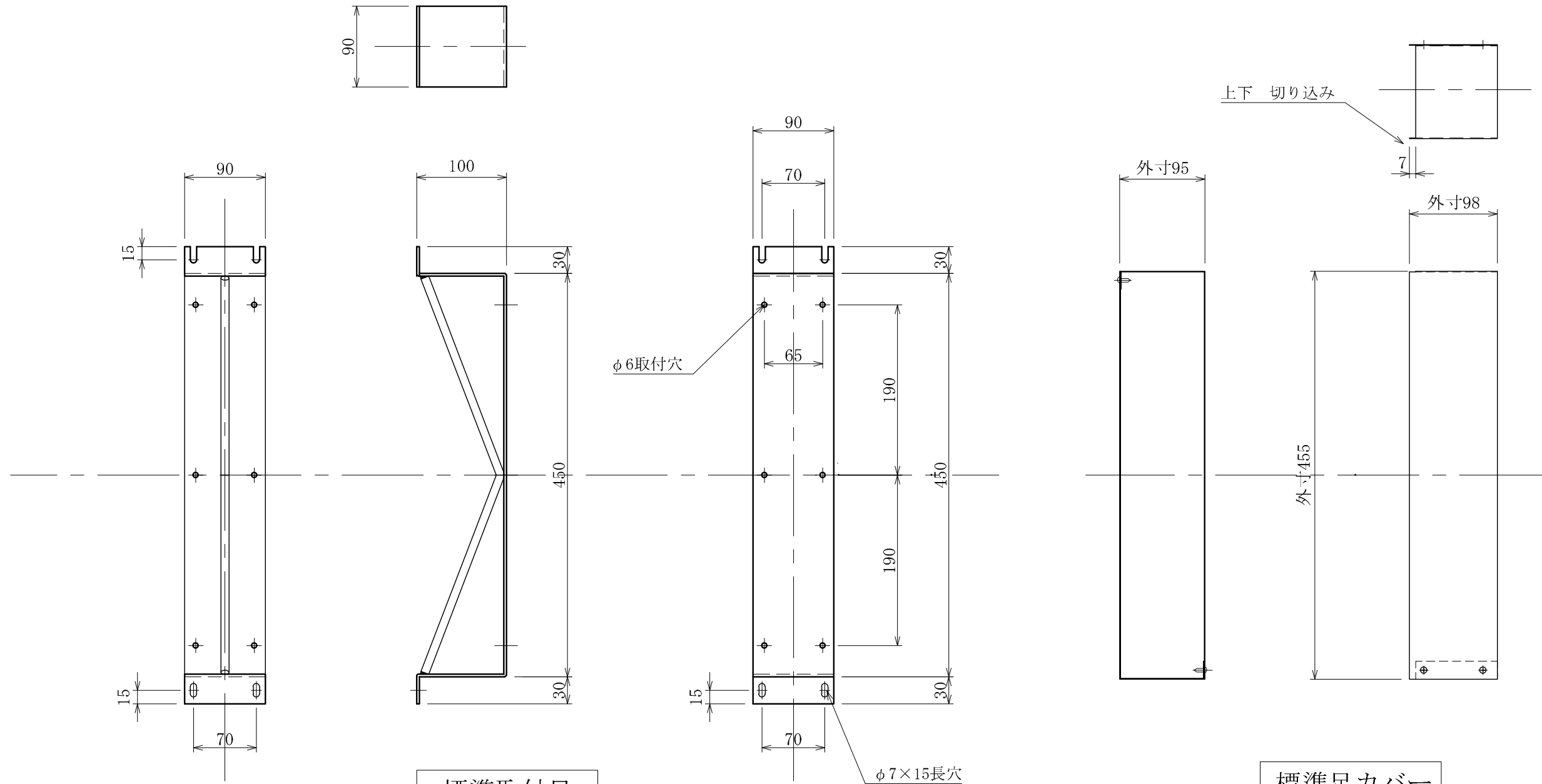
標準取付足 スチール
