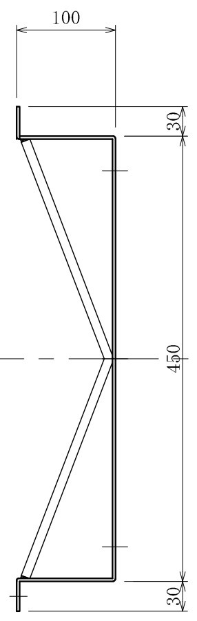
標準取付足 スチール
