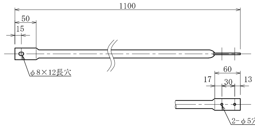
標準取付足 スチール
